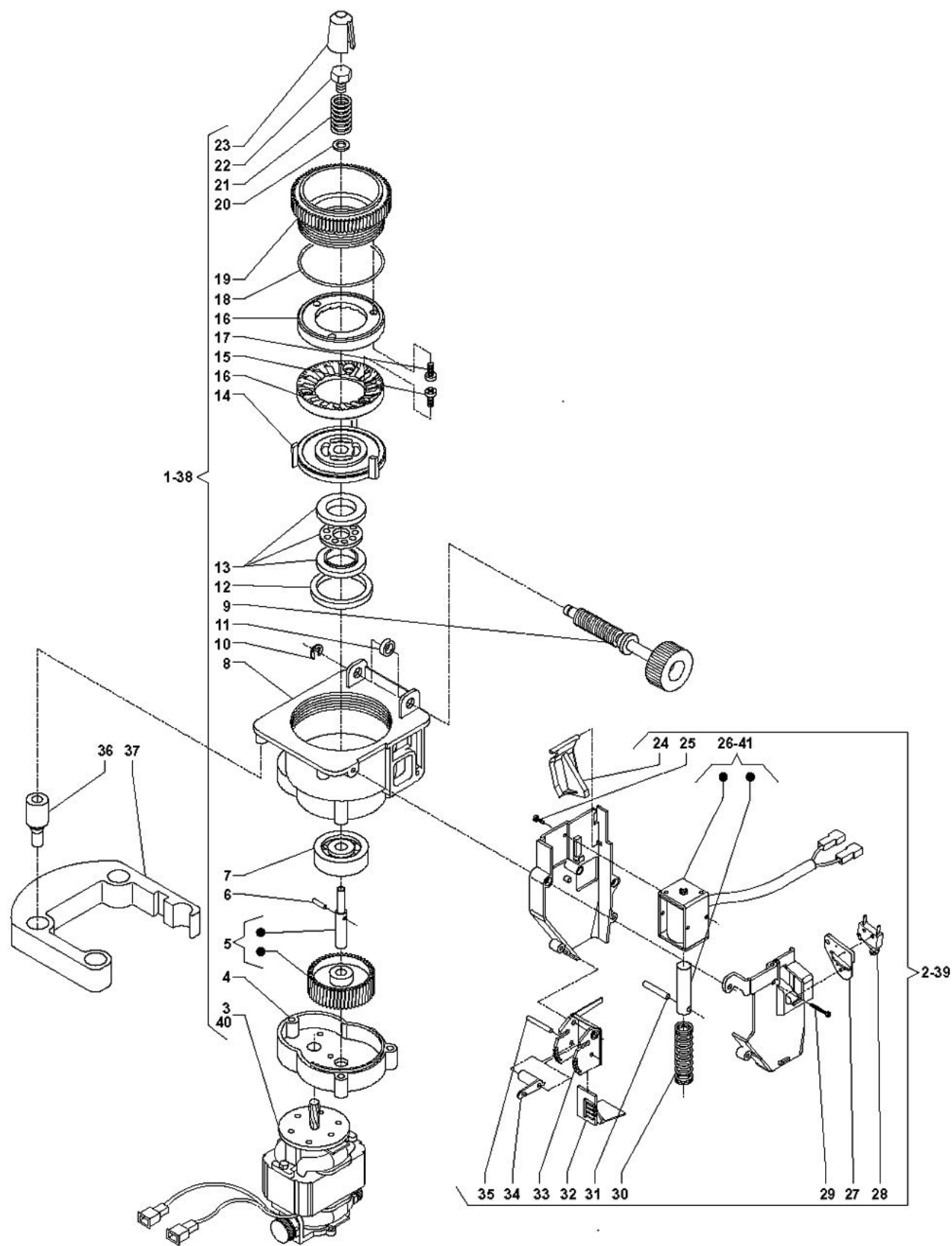
Tavola :08 - Macinadossatore
