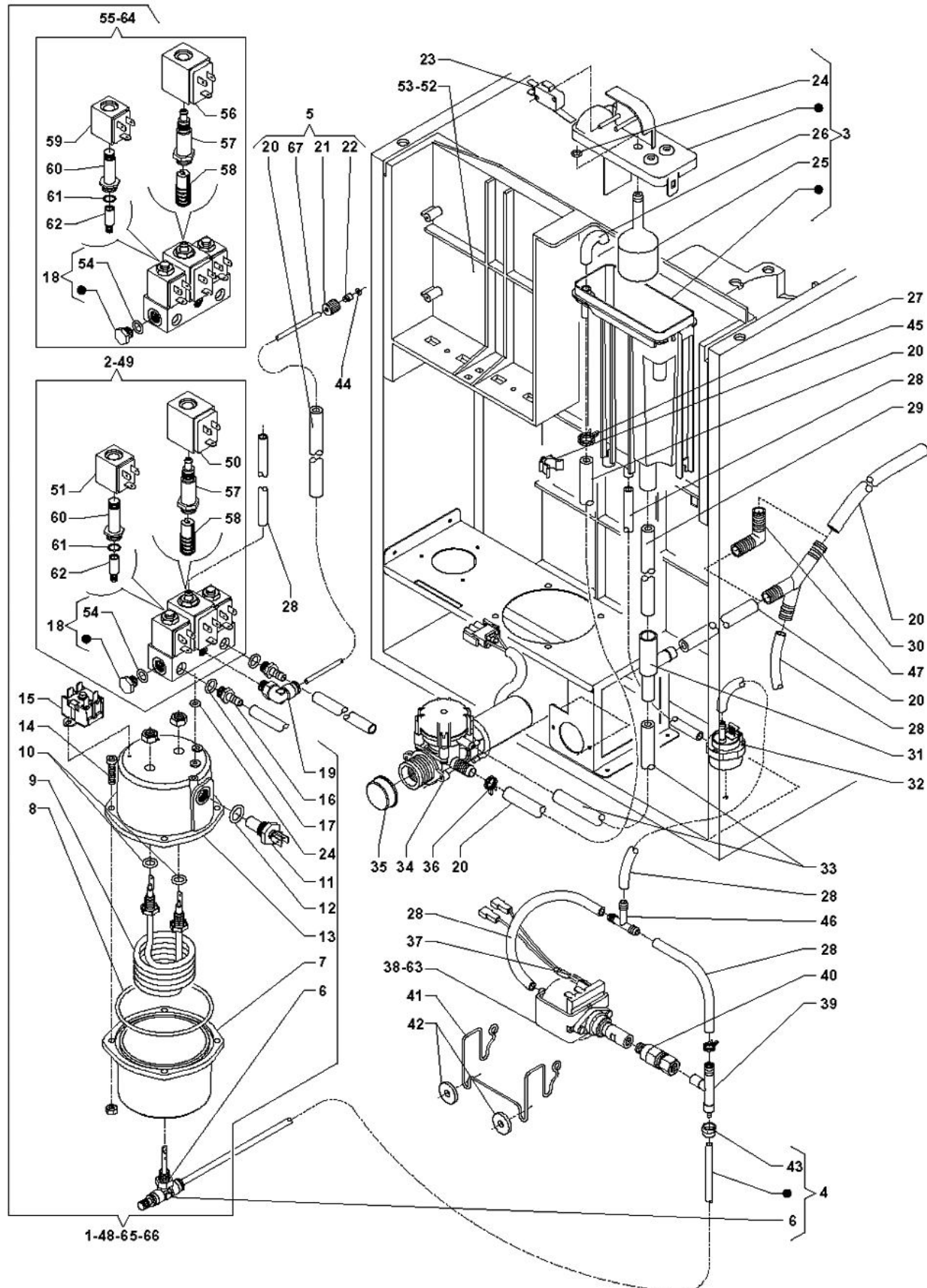
Tavola :04 - Circuito idraulico
