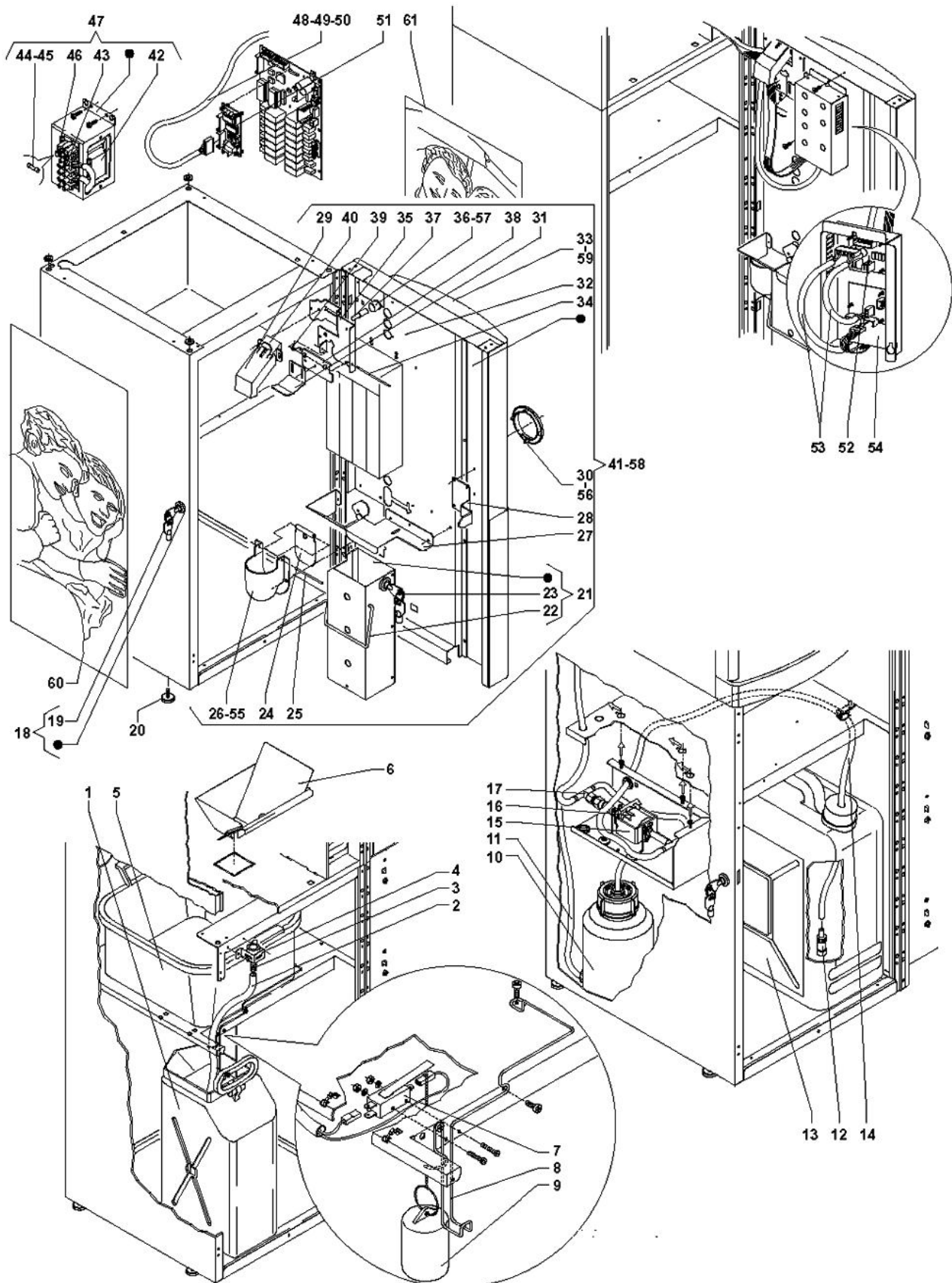
Tavola :10 - Mobilietto e kits
