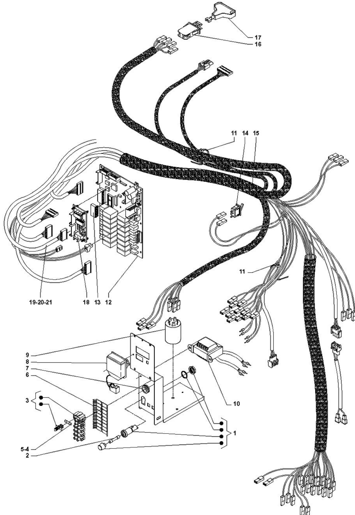
Tavola :03 - Impianto elettrico
