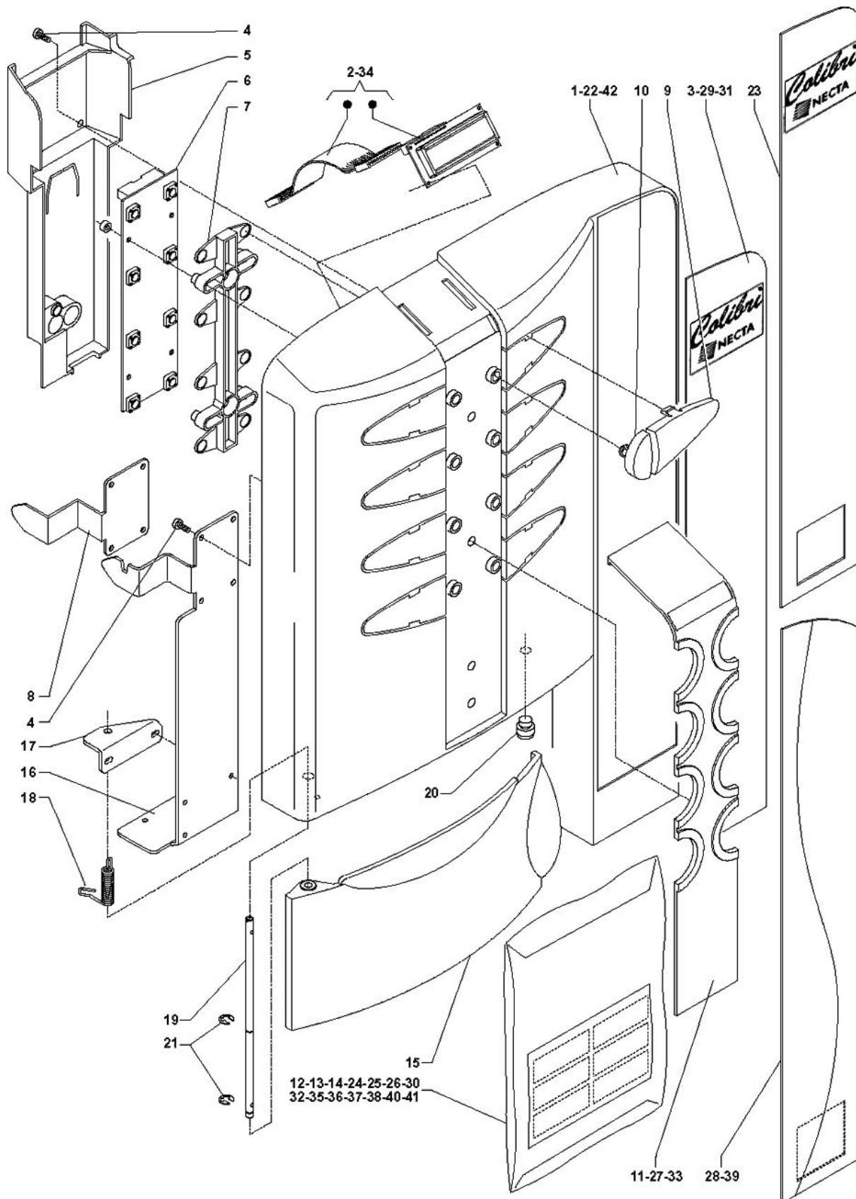
Tavola :01 - Porta
